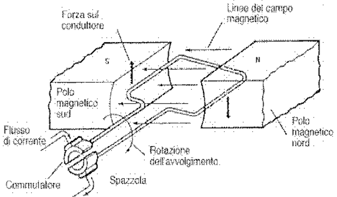
Struttura di base di un motore D.C.
